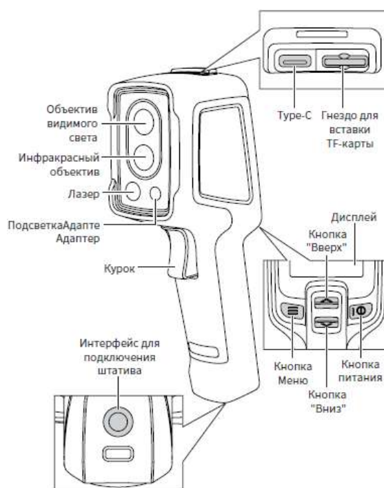
Рис. 2. Устройство тепловизора
