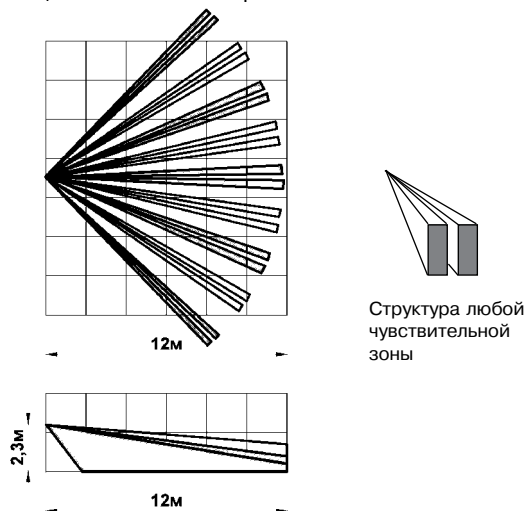
Рисунок 1 – Диаграмма зоны обнаружения
