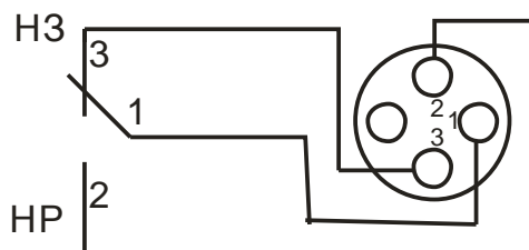
Рисунок Б.2 - Исполнение с разъемом
